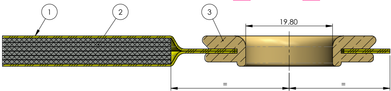
SECTION A-A SCALE 2 : 1
